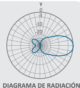
DIAGRAMA DE RADIACIÓN
