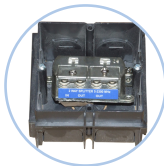
Instalación en caja de mecanismos
